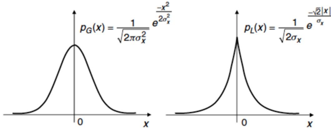
Gaussian PDF
